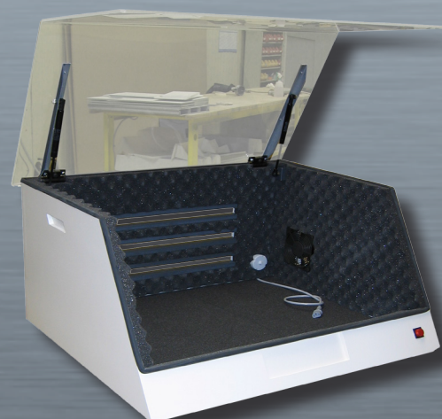
CAJA DE INSONORIZACIÓN abierta con vista sobre las salidas del papel en la parte trasera
